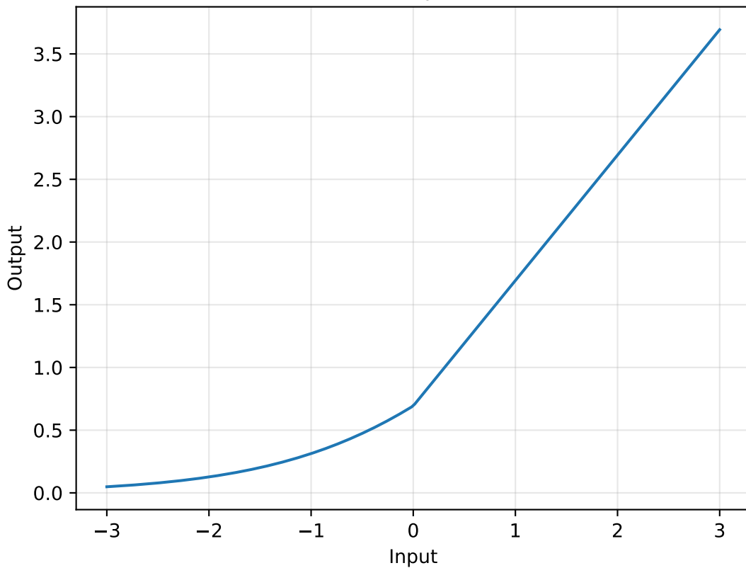
Rectified Softplus (ReSP)
